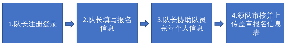
图1 报名流程图
