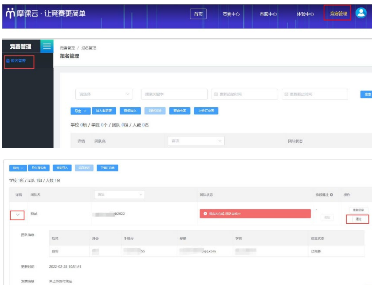
图13 报名审核
